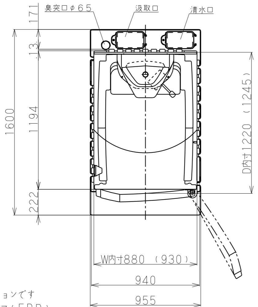
平面図
