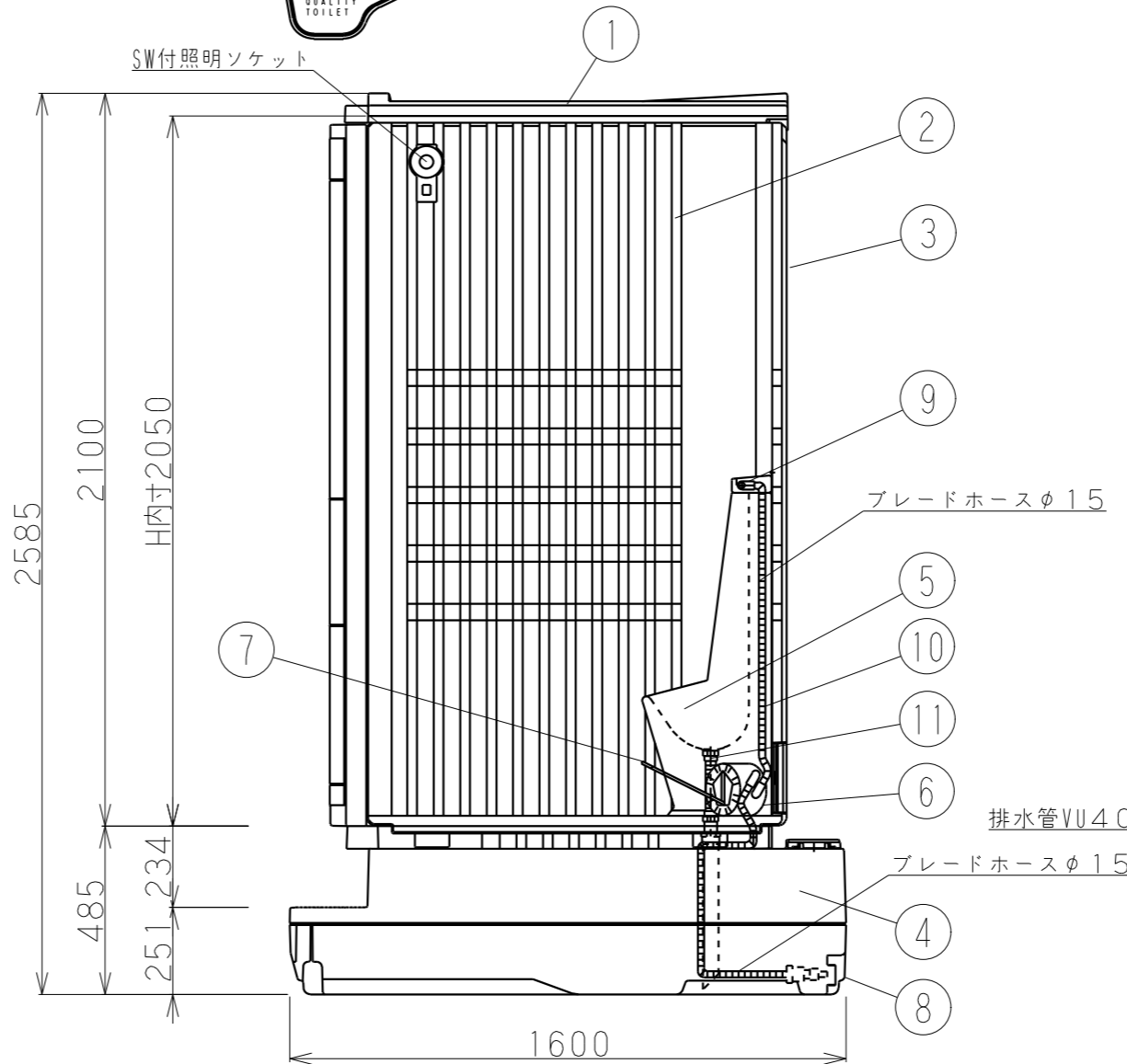
側面図
