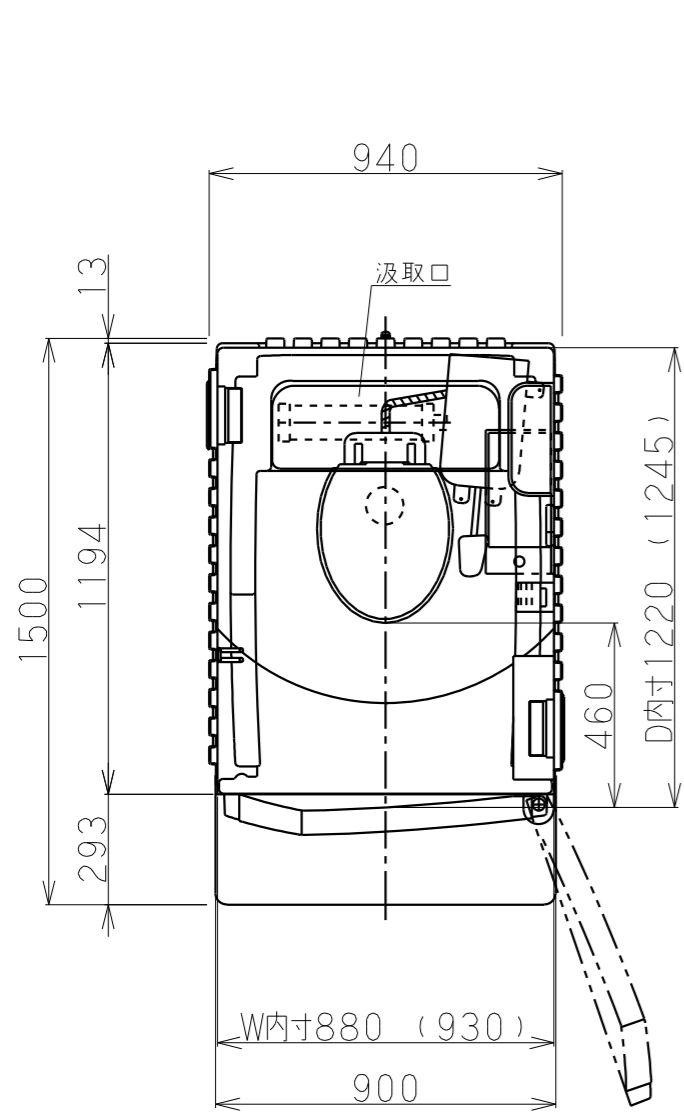
平面図
