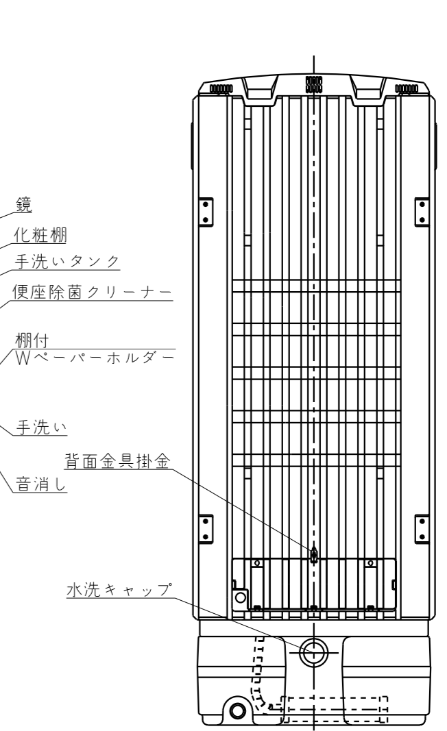
背面図
