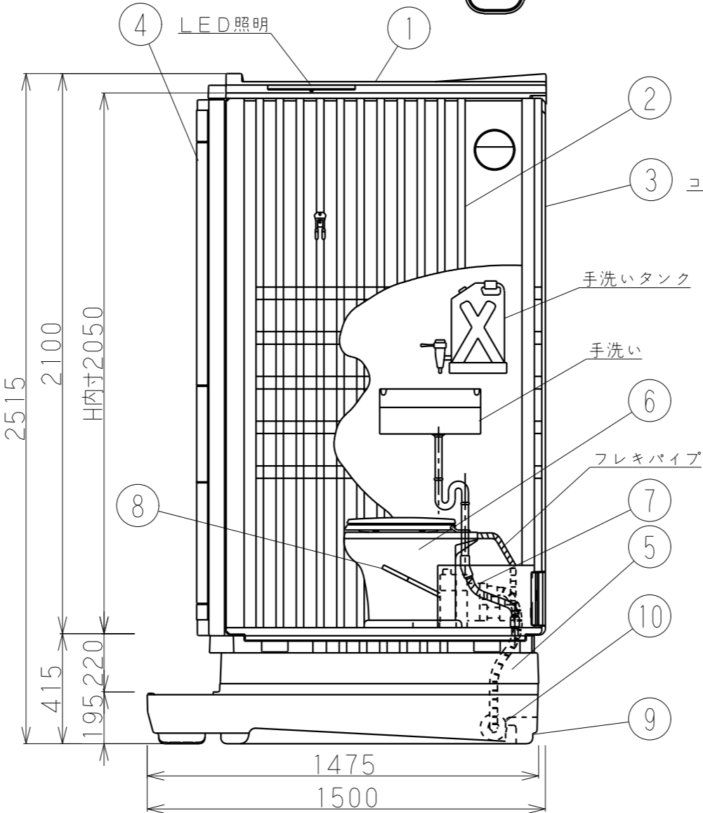
側面図
