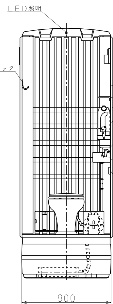
正面図
