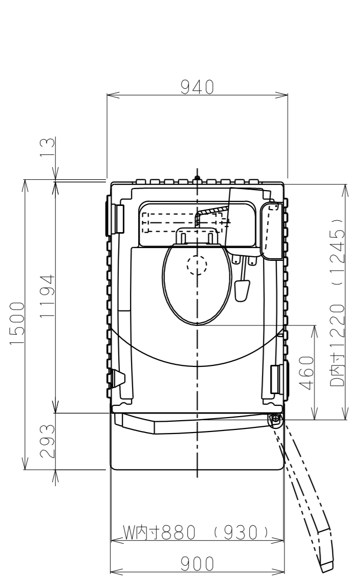
平面図
