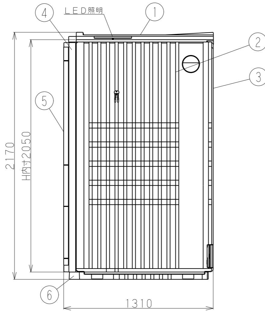
側面図
